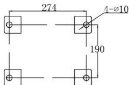
安装尺寸
