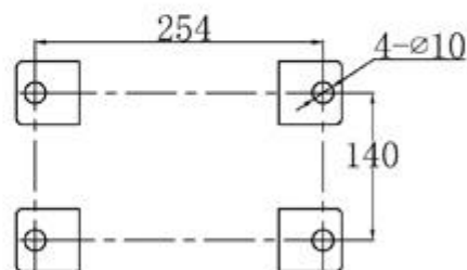
安装尺寸
